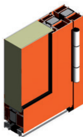
Querschnitt EUROA 90 Tür Aufsatzfüllung einseitig Dicke 83 mm.
